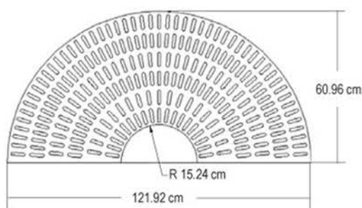
CITYGRATE44R
