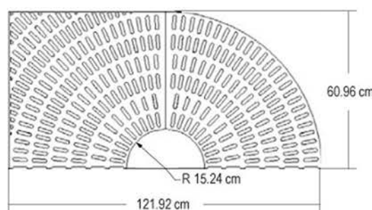
CITYGRATE44RC
