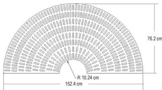
CITYGRATE55R
