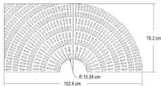
CITYGRATE55RC
